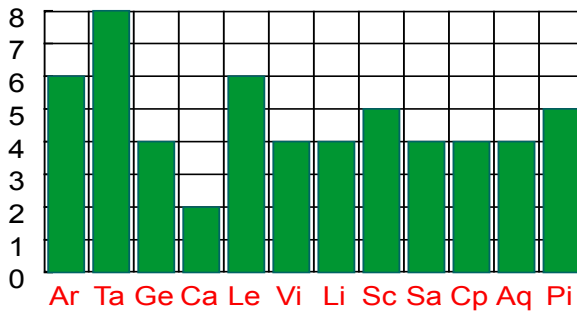
Jupiter
