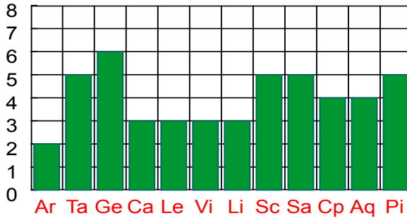
Mars
